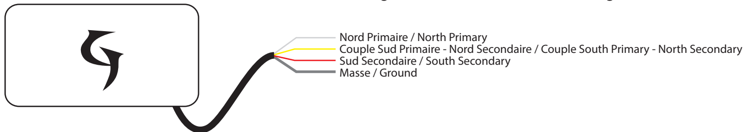
Câblage Humbucker / Humbucker Wiring
